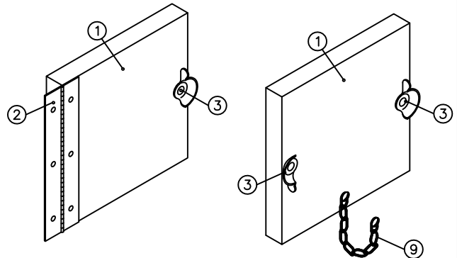
FSA125SM: HINGED DOOR
