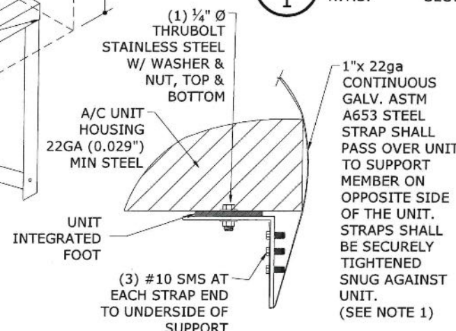
5 STRAP DETAIL 1 N.T.S. SECTION VIEW
